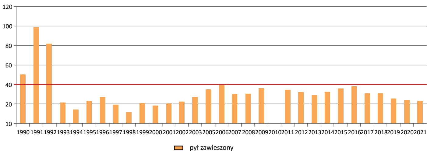
Wykres 8.1. Wieloletnie wyniki pomiarów zanieczyszczeń PM10 na terenie Dzierżoniowa
